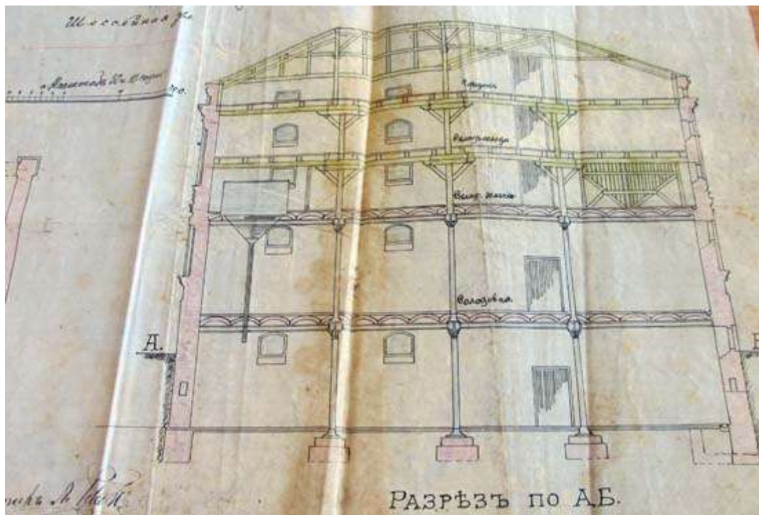
Креслення одного з цехів
