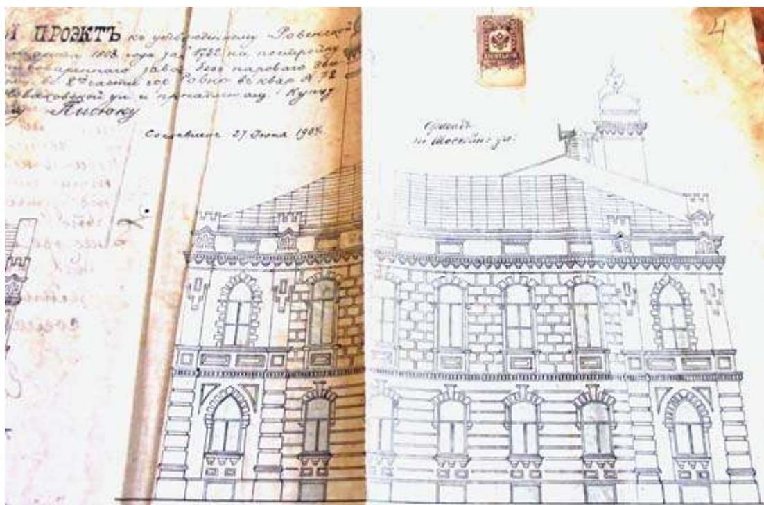
З того Додаткового проекту - фасад будівлі з вулиці Шосової (Соборної)
